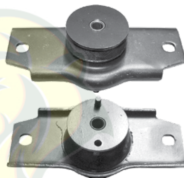
N° AMASA 9634 OE # 96340027 APLICACIÓN. SOPORTE CAJA DE VELOCIDADES MATIZ G2 1.0 STD MOD. 03/08
