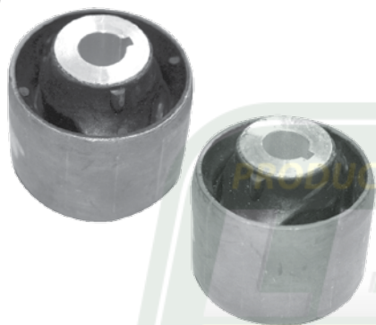
N° AMASA VW 182-A OE # 7H0407182A APLICACIÓN. BUJE HORQUILLA EUROVAN T5 DIESEL TRASERO MOD. 2005/UP
