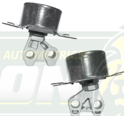
N° AMASA 02282 OE # 93302282 APLICACIÓN. SOPORTE TRANSMISIÓN CORSA MOD. TODOS
