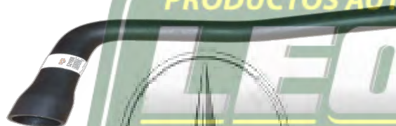
521908 Ø INT. 45mm Ø INT. ANCHO 58mm RADIADOR INFERIOR
