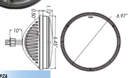
LUZ :ALTA Y BAJA PZA 20 PZAS X CAJA UNIDAD 7" CON 36WATTS DE POTENCIA CM-7070
