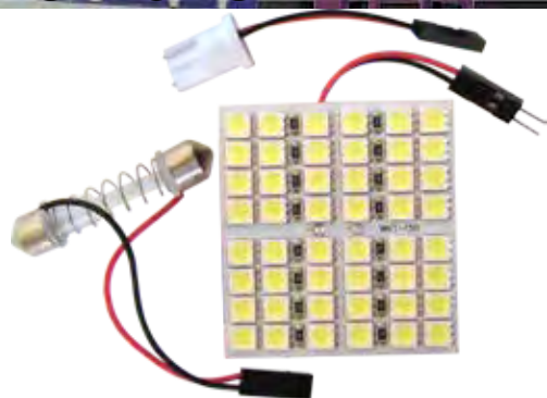
200 JGOS X CAJA MEDIDA: 50MM X 46MM LUZ PARA DOMO 48 LEDS CON ADAPTADORES 138-48SMD 48 X 5050SMD
