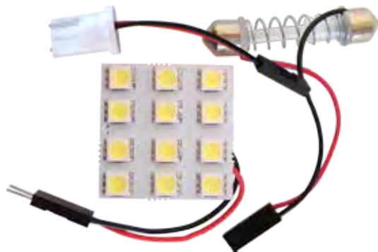
200 JGOS X CAJA MEDIDA: 30MM X 30MM LUZ PARA DOMO 12 LEDS CON ADAPTADORES 12SMD-5050 12 X 5050SMD
