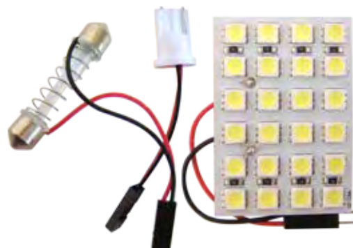
200 JGOS X CAJA MEDIDA: 50MM X 35MM LUZ PARA DOMO 24 LEDS CON ADAPTADORES 137-24SMD 24 X 5050SMD
