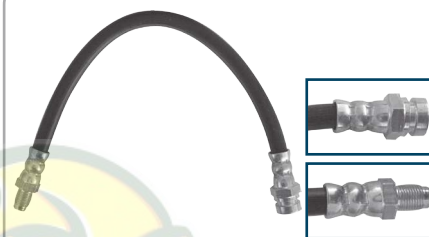
N° AMASA LC-1204 REF BH38125 APLICACIÓN. Nissan 83/87 Samurai; 87/88 200SX; 74/77 710; 80/86 720; 86 D21. Datsun 79/82 Trasera MOD. 1974/88
