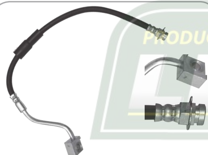
N° AMASA LC38899 REF: BH38899, 124725, bh178170 APLICACIÓN. Ford Cta. Bronco USA F150 Delantera Derecha MOD. 1990/ 96
