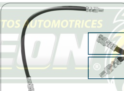
N° AMASA LC-1212 REF BH36736 APLICACIÓN. Nissan 69/73 510; 72/74 610; 74/75 710; 79/82 310; 76/78 F10; 87/89 Van. Datsun Delantera Der-lzq. MOD. 1969/89
