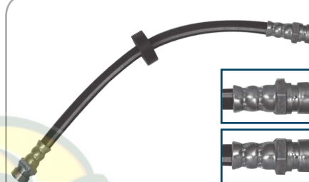
N° AMASA LC-38840 REF: BH38840, 124718 APLICACIÓN. Escort F. Tambor Auto. Trasera-Der-Izq MOD. 1994/00
