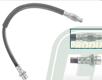
N° AMASA LC-1179 REF BH36699/78092/80957 APLICACIÓN. Fairmont, Maverick, Galaxie Auto, Delantera-Der-Izq MOD. 1974/81
