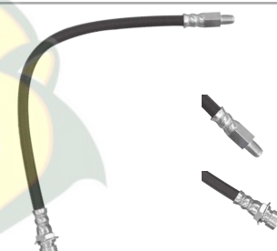
N° AMASA LC1184 REF: BH3681471344/80023 /86582 APLICACIÓN. Ford B-600, F-600 Cta Trasera MOD. 1980/85
