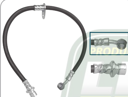
N° AMASA LC-382559 REF BH382559 APLICACIÓN. Honda 07-09 CR-V Delantera Derecha MOD. 2007/09
