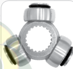
21211 21 Dientes, 1.178 MED REF.: 327747 RT-2995 Renault 5 Isuzu I
