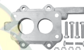
6059 Base de carburador Serie K. Motor 135 2.2 L. y 2.5 L. de 1982/88 Sin Tubo de vacio Con tornillos y junta No. Original: 4293755
