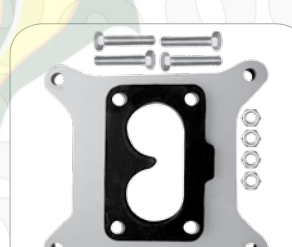
B-305A Adaptación Ford/Chev. o Dodge Holley 4 a 2 g. Con tornillos y junta
