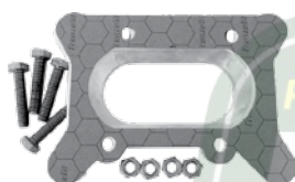
12-38 Conversión Dodge TBI 2 gargantas a Ford 2 gargantas motorcraft Microbus 92 Pick-Up importada, Ram-Charger Con tornillos y junta
