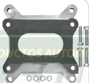
12-18 Conversión Ford Todos V-8 de 4 gargantas a 2 gargantas - Motorcraft Con tornillos y junta
