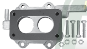
6059-A Base de carburador Serie K. Motor 135 2.2 L. y 2.5 L. de 1984/90 Con Tubo de vacio. Con tornillos y junta No. Original: 4300988
