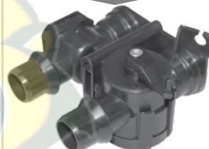
V-69686 Ref.: V-9686 Válvula control circulación de aire caliente Chevy Corsa 1.8L 4 Cil. 00/07 No. Original: 93369686
