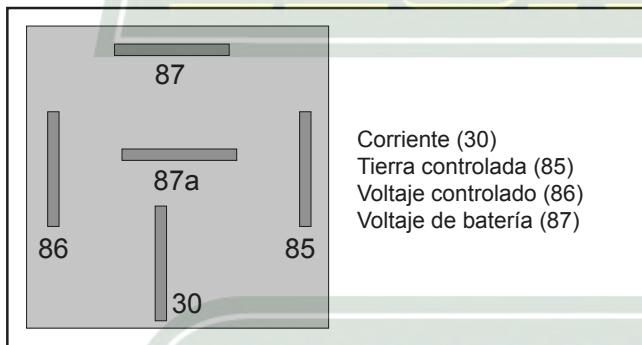
Relevador
