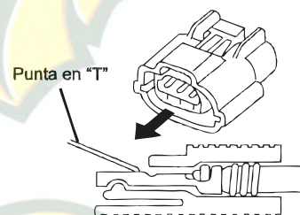
Terminal hembra
