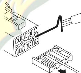
Seguro conector
